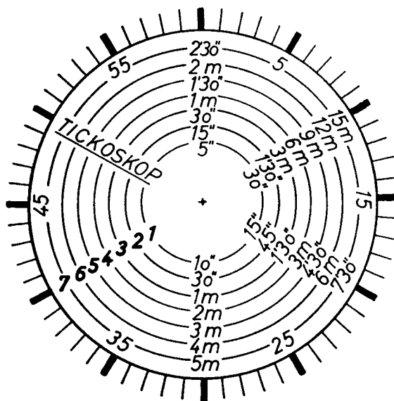
Abbildung 2: Spezialzifferblatt für Tickoskop
